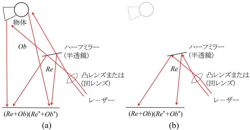
図 2.1 (a) ホログラム撮像時の光学系と (b) ホログラム再生時の光学系。「ポジ」の乾板に干渉像が記録される
