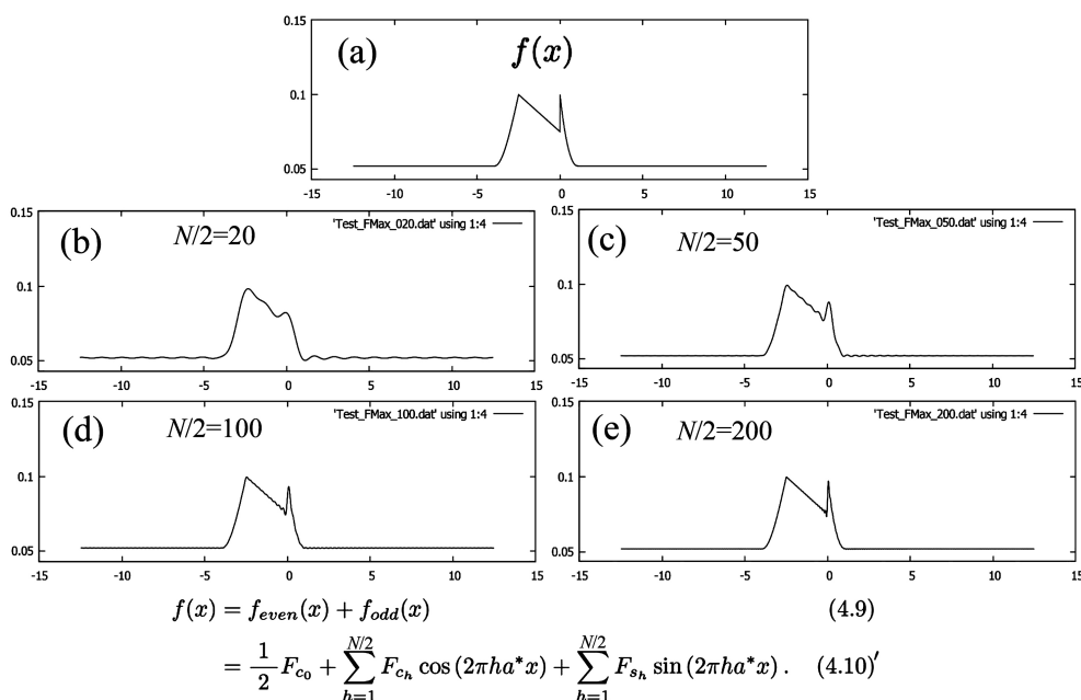
図 4.5 (a) もとの関数。式 (4.10) [p.23] で \infty の代わりに, (b) N/2 = 20 , (c) N/2 = 50 , (d) N/2 = 100 , (e) N/2 = 200 の有限な範囲でサンメーションを打ち切った級数による計算値
