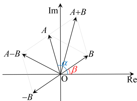
図 1.3 複素数の足し算と引き算は、2次元のベクトルと同様におこなわれる
