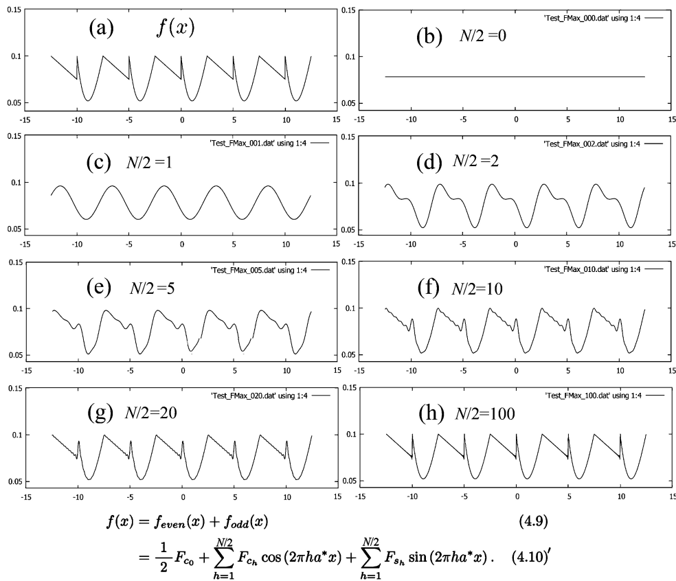
図4.3 (a) もとの関数。式(4.10) [p.23] で \infty の代わりに, (b) N/2 = 0 , (c) N/2 = 1 , (d) N/2 = 2 , (e) N/2 = 5 , (f) N/2 = 10 , (g) N/2 = 20 , (h) N/2 = 100 の有限な範囲でサンメーションを打ち切った級数による計算値
