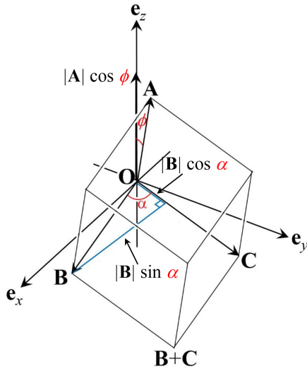
図 B.5 \mathbf{A} , \mathbf{B} , \mathbf{C} のスカラー三重積はこれらのベクトルを稜とする平行六面体の体積である。図 5.3 [p.55] の再掲
