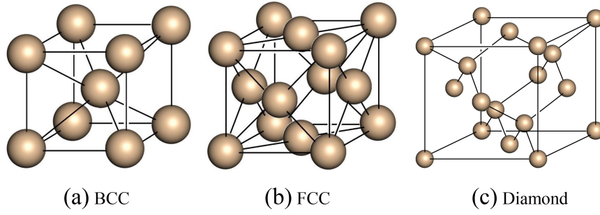
図 9.2 (a) 体心立方格子, (b) 面心立方格子, (c) ダイヤモンド型格子の原子配列
