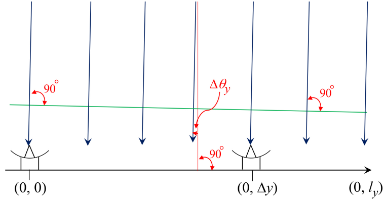
図 6.4 (0, 0) と (0, Δy) の位置に並んだ 2 つのパラボラアンテナで構成される電波干渉計。右のアンテナは Δy 方向に可動であるとする
