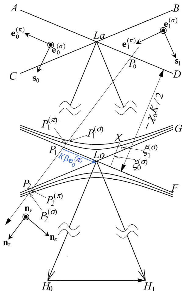
図 K.1 逆空間に作図した分散面。ブロッホ波の波数ベクトル始点は、ローレンツ点 L_0 で交差する近似的直線 P_1F および P_2G を漸近線とする双曲線上になければならない。 P_1 直上にある P_1^{(\sigma)} , P_1^{(\pi)} を通る双曲線は、 \sigma 偏光と \pi 偏光に対する分散面である
